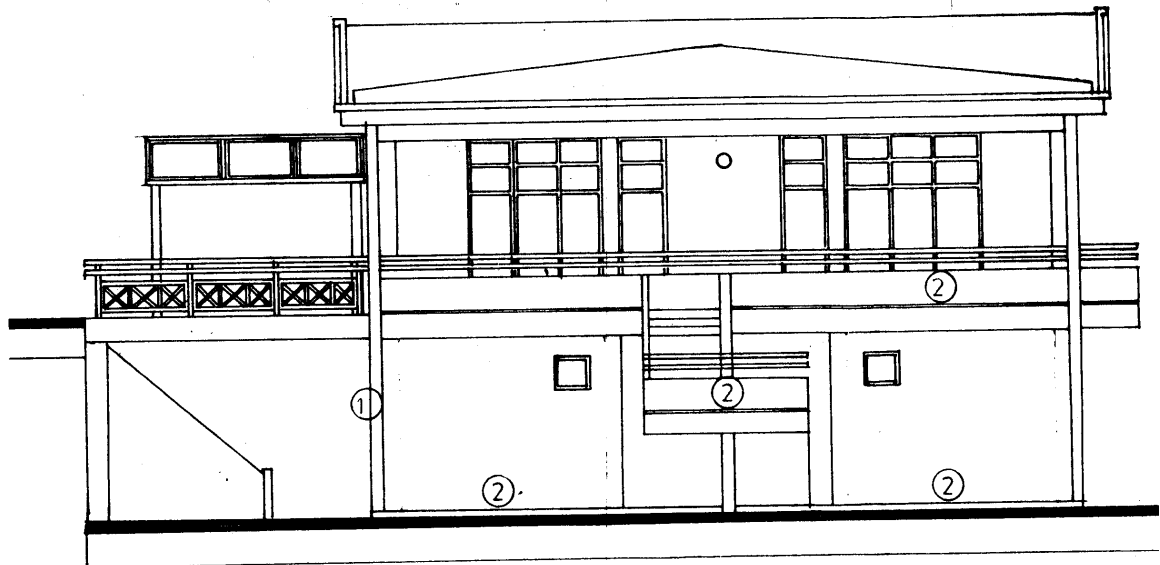
ЕРО • ЗАПАДЕН ИЗГЛЕД М - WEST ELEVATION 1:100
