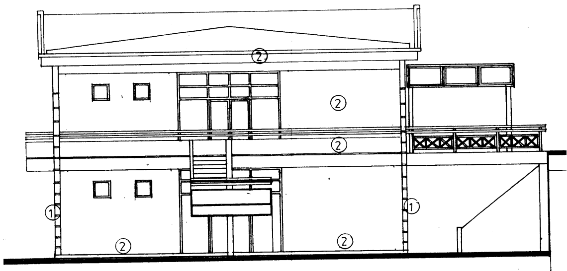
• ИСТОЧЕН ИЗГЛЕД М1: EAST ELEVATION 1:100
